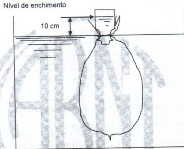
Figura 2 — Sistema de amarração para o fechamento
